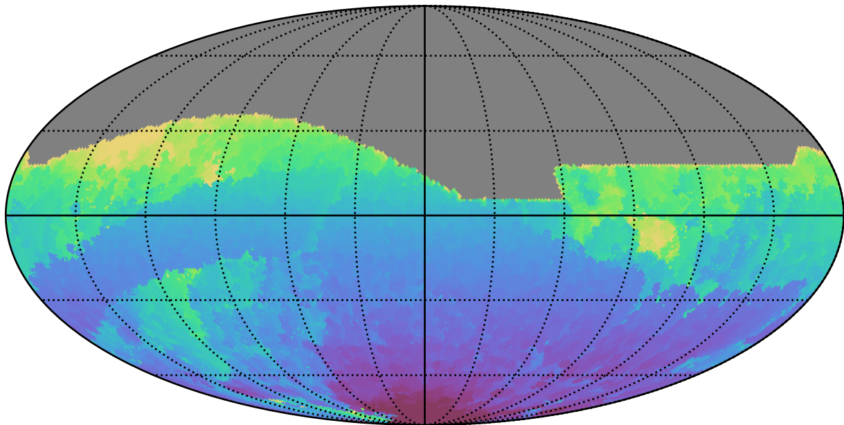
weather_cloudso35v3.4_10yrs All sky r band: Min HA
