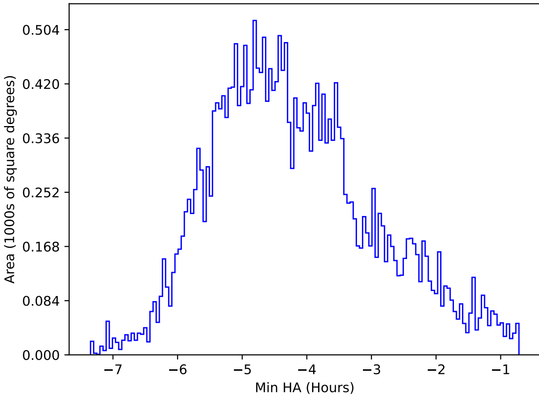
weather_cloudso35v3.4_10yrs All sky r band: Min HA
