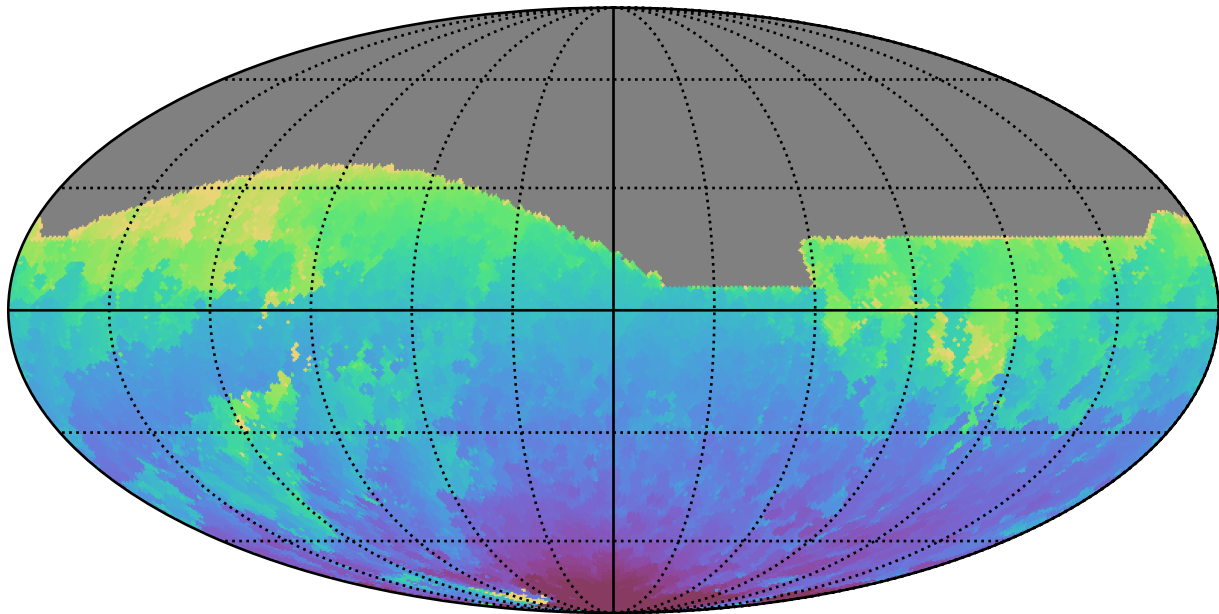
weather_cloudso35v3.4_10yrs All sky i band: Min HA
