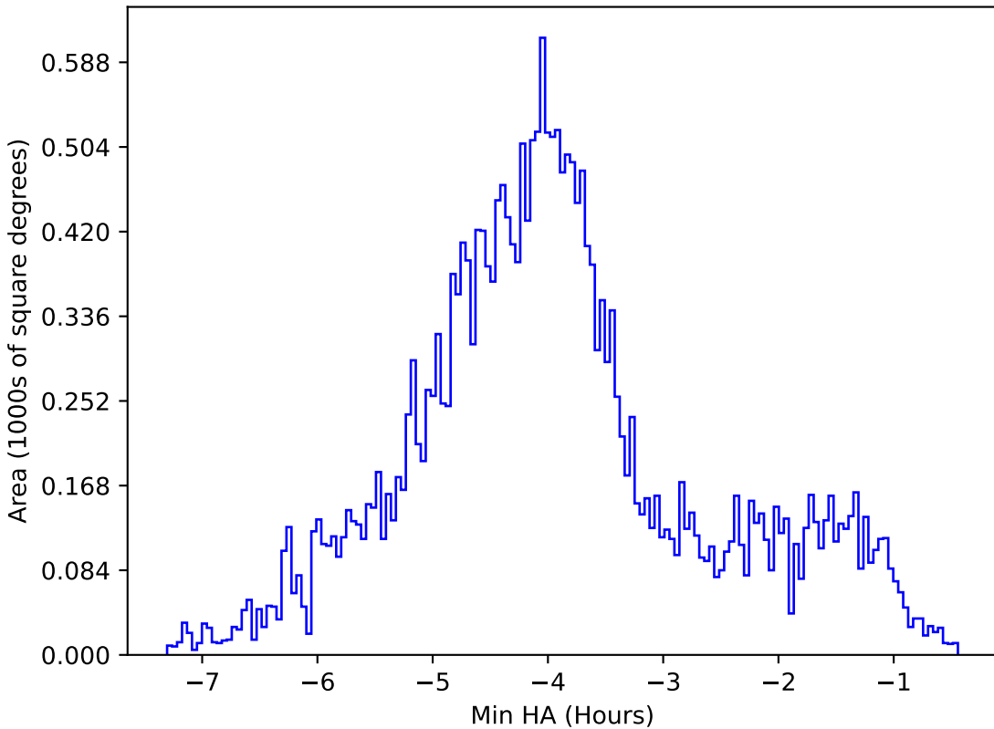
weather_cloudso35v3.4_10yrs All sky g band: Min HA
