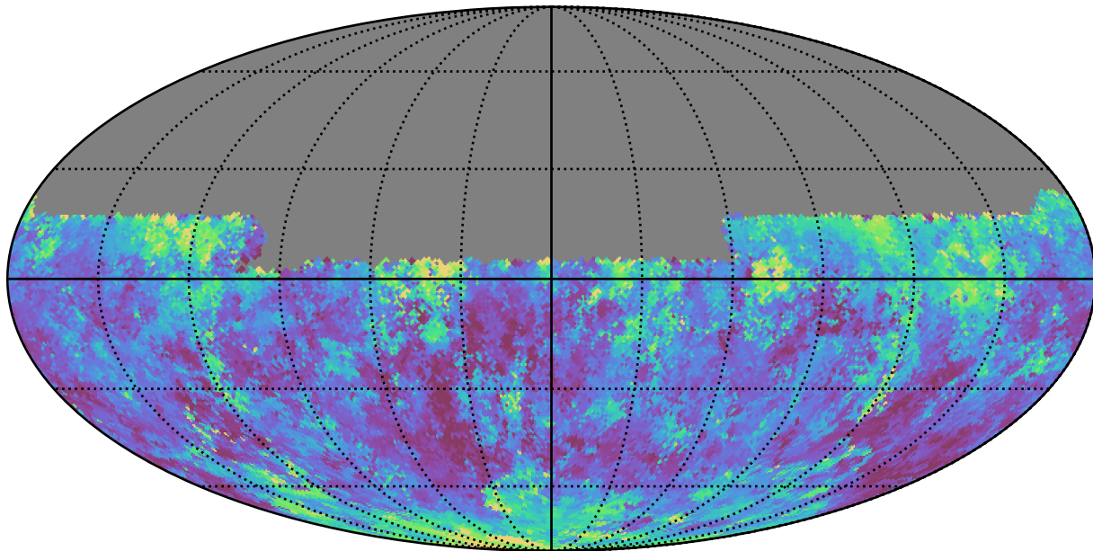
weather_cloudso35v3.4_10yrs Yr 1 y band: Median seeingGeom
