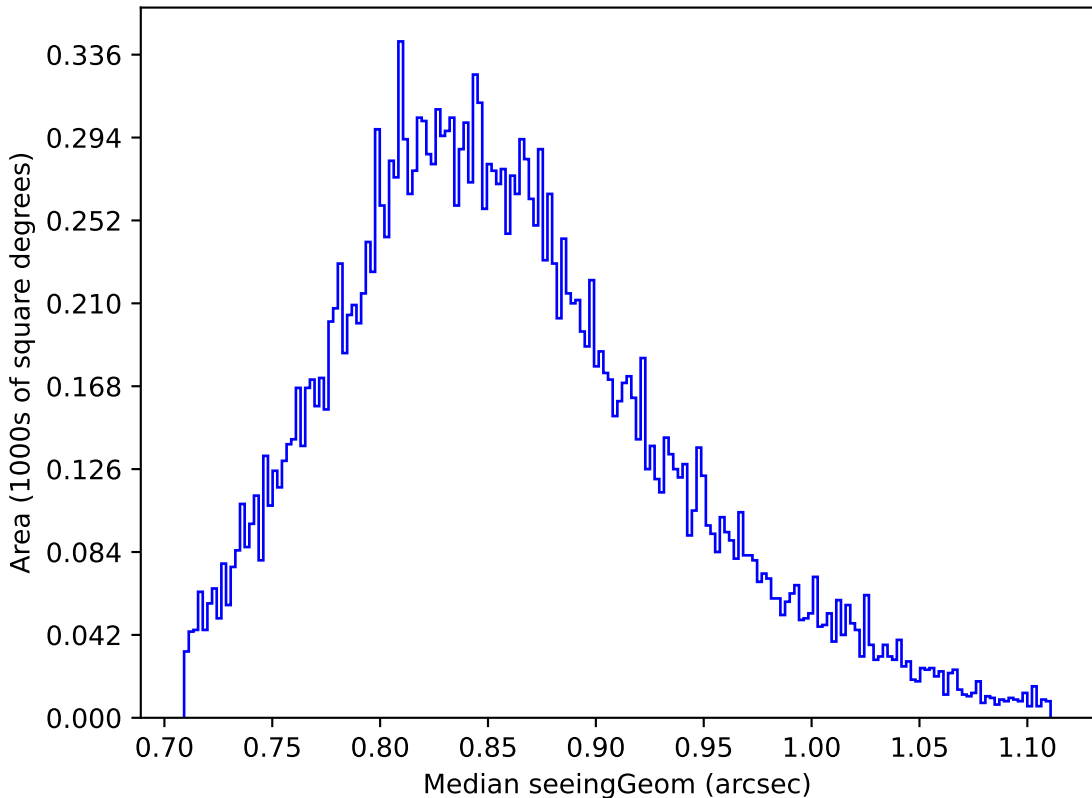
weather_cloudso35v3.4_10yrs Yr 1 y band: Median seeingGeom
