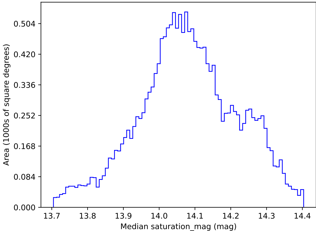
weather_cloudso35v3.4_10yrs WFD z band: Median saturation_mag
