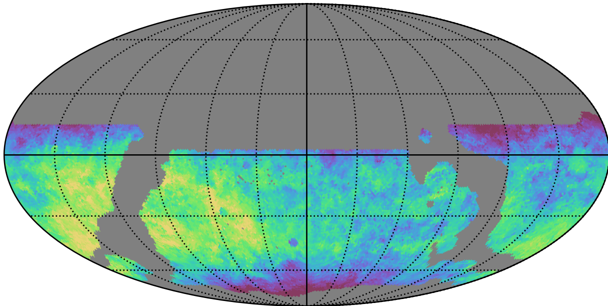
weather_cloudso35v3.4_10yrs WFD y band: Median saturation_mag
