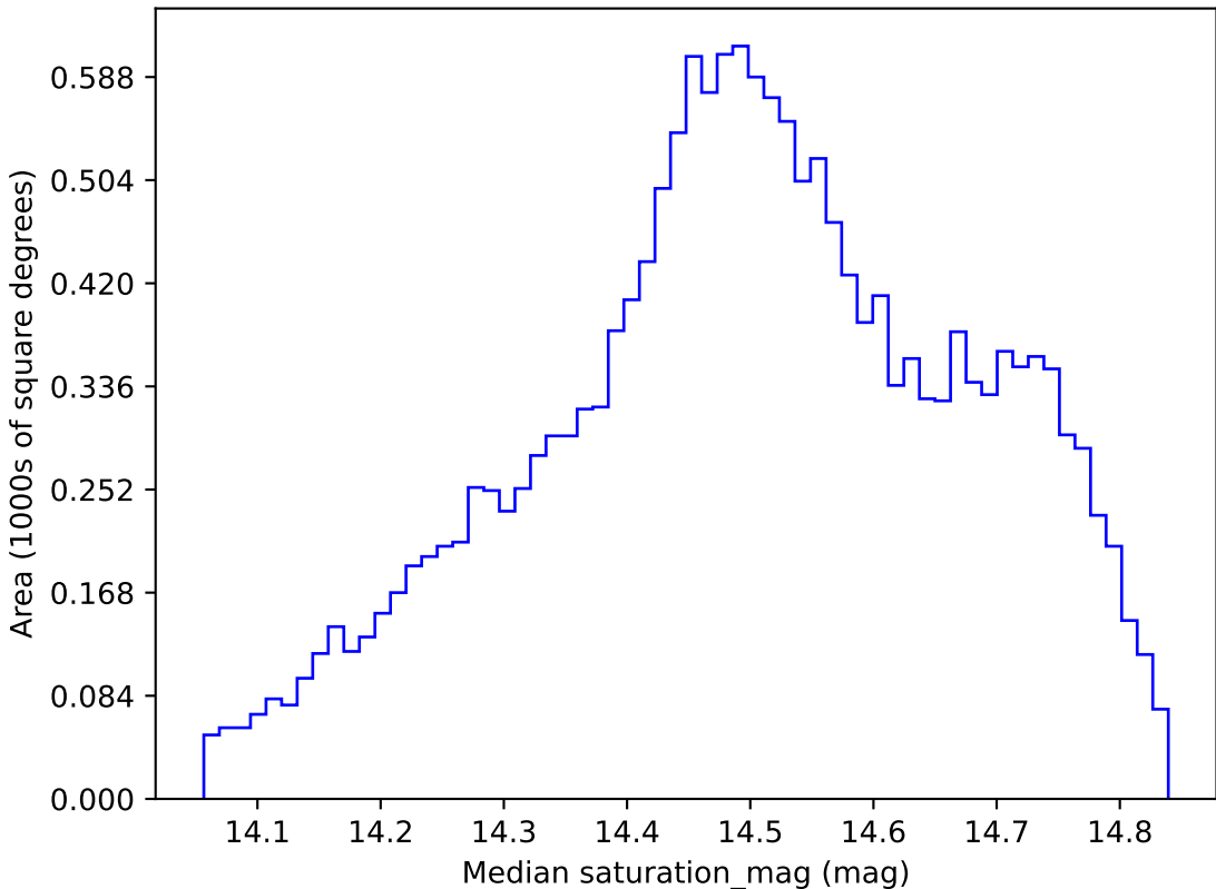
weather_cloudso35v3.4_10yrs WFD i band: Median saturation_mag
