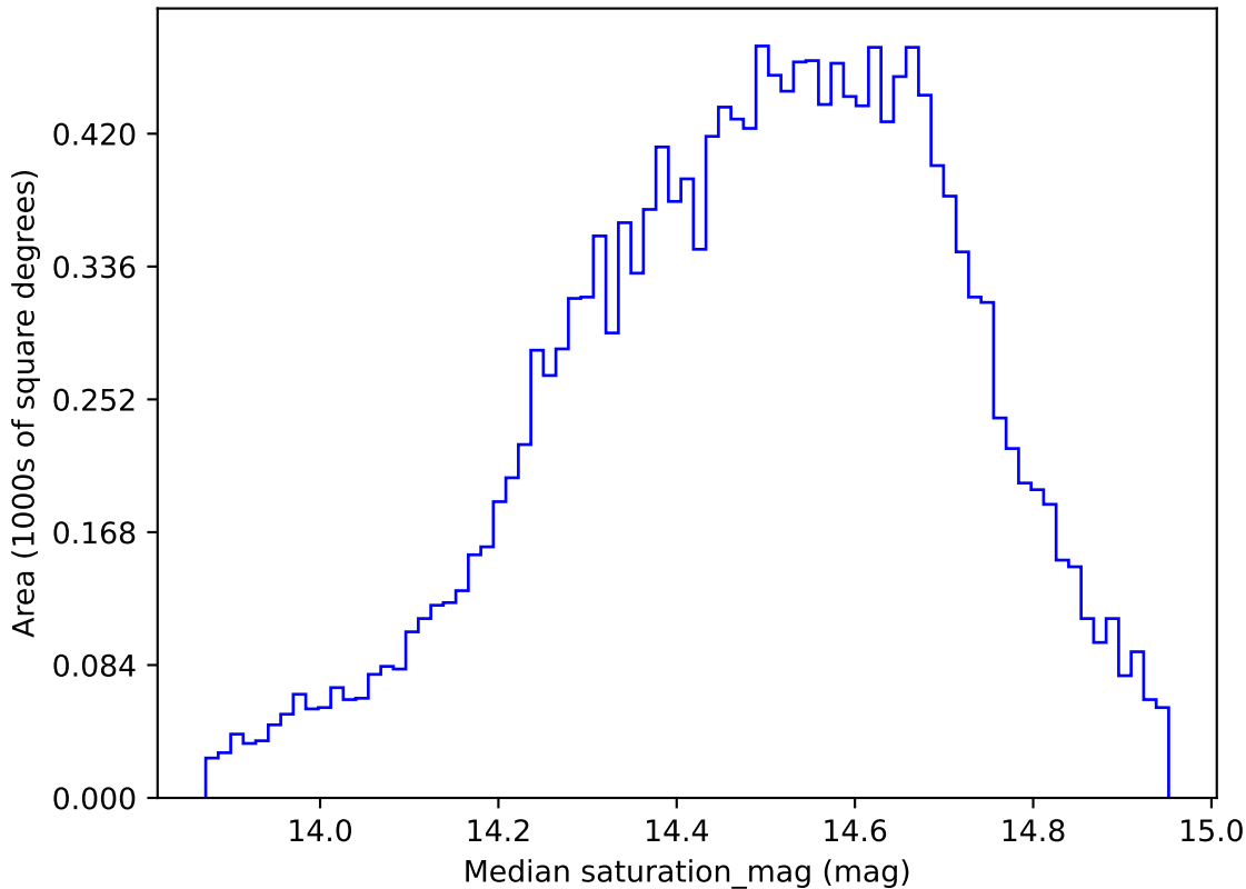
weather_cloudso35v3.4_10yrs WFD g band: Median saturation_mag
