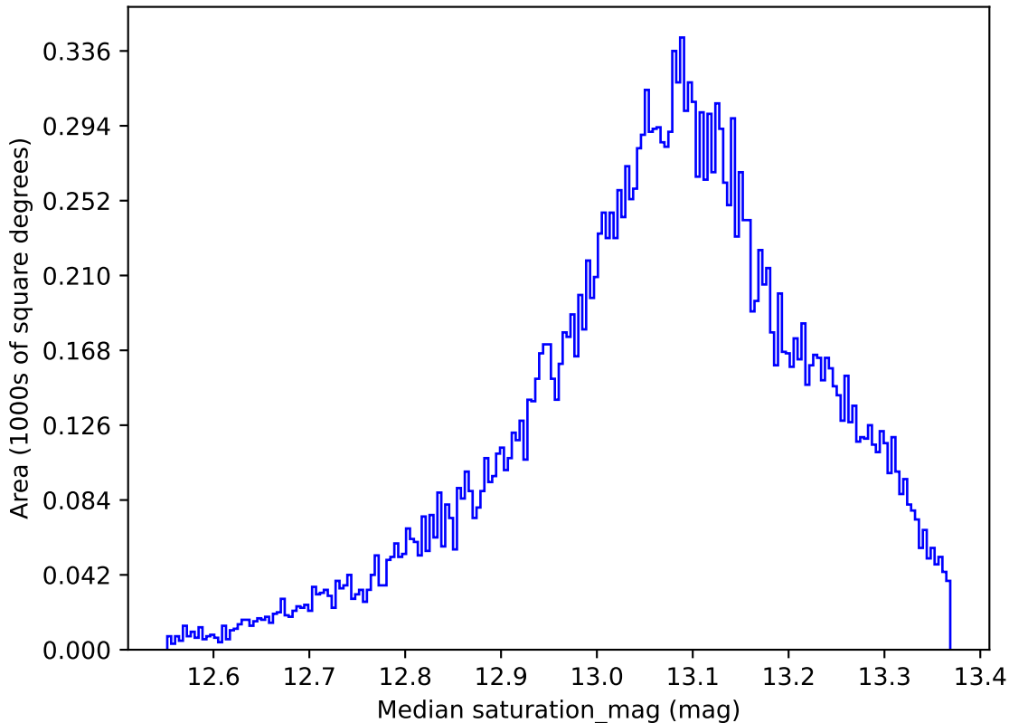
weather_cloudso35v3.4_10yrs All sky y band: Median saturation_mag
