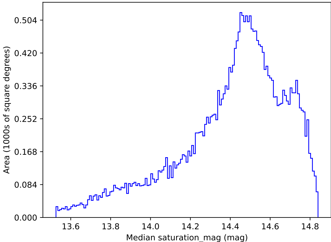
weather_cloudso35v3.4_10yrs All sky i band: Median saturation_mag
