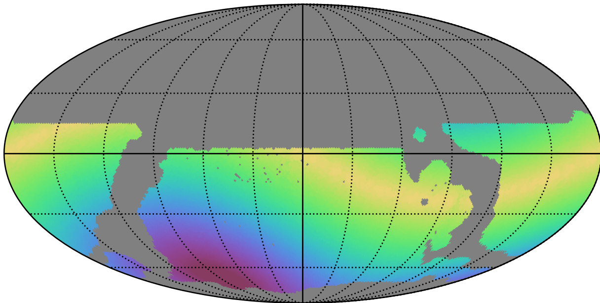
weather_cloudso35v3.4_10yrs WFD y band: Max solarElong
