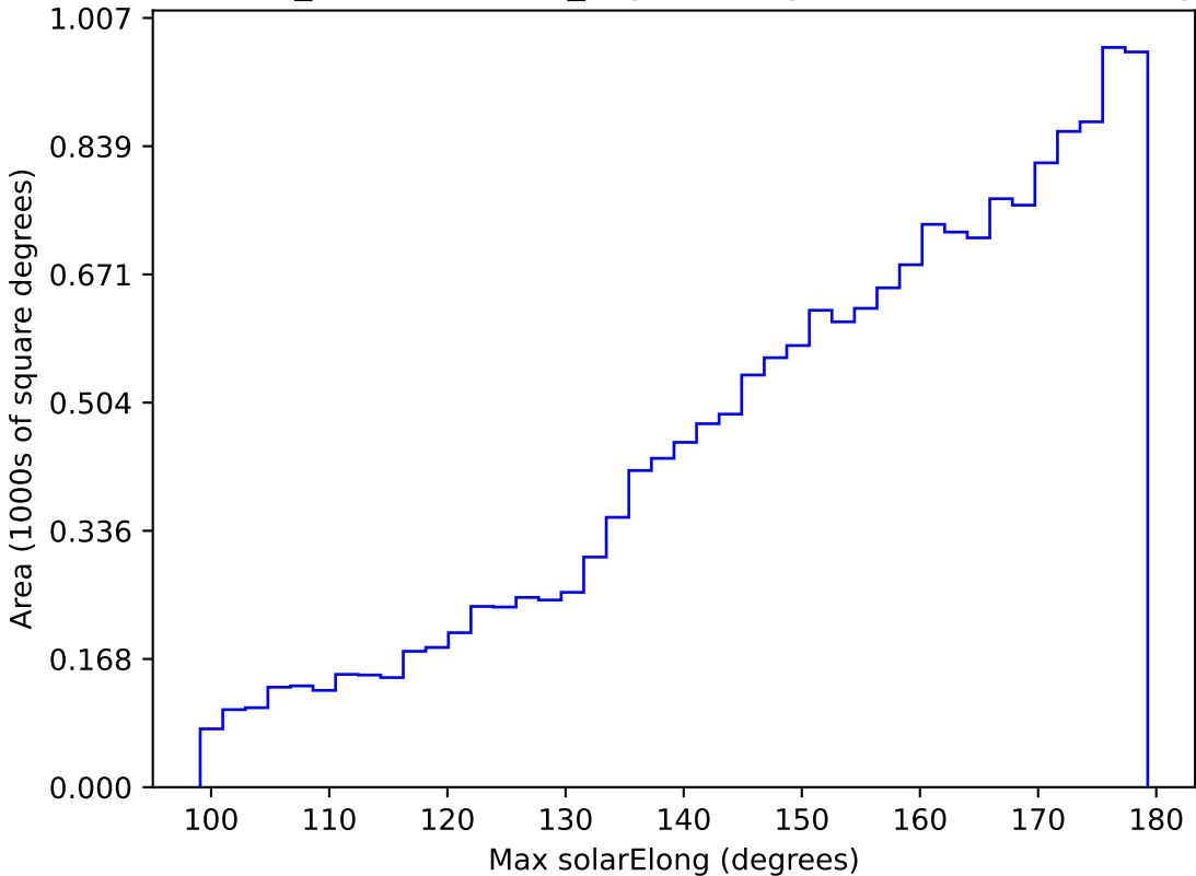
weather_cloudso35v3.4_10yrs WFD y band: Max solarElong
