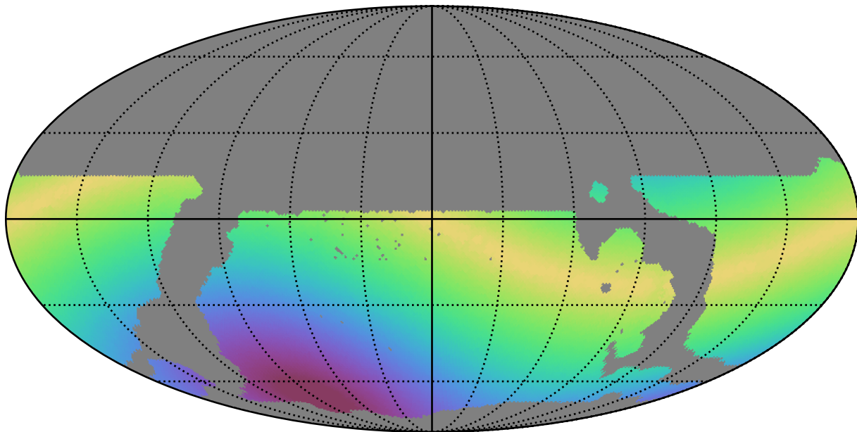
weather_cloudso35v3.4_10yrs WFD i band: Max solarElong
