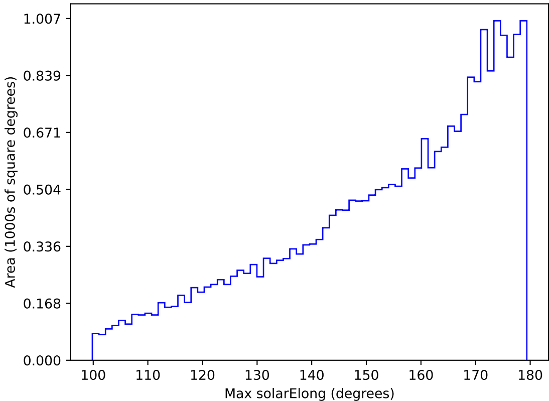
weather_cloudso35v3.4_10yrs All sky i band: Max solarElong
