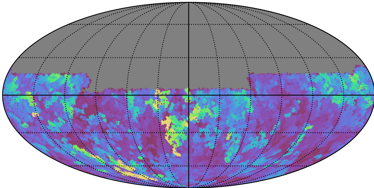
weather_cloudso35v3.4_10yrs Yr 1 y band: Max seeingGeom
