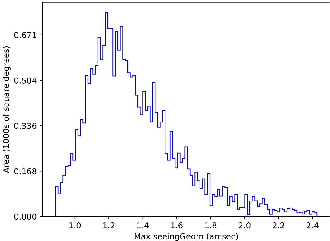
weather_cloudso35v3.4_10yrs Yr 1 y band: Max seeingGeom
