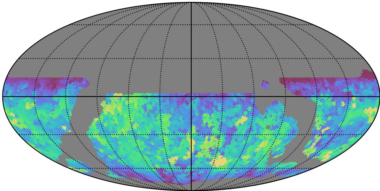
weather_cloudso35v3.4_10yrs WFD z band: Max saturation_mag
