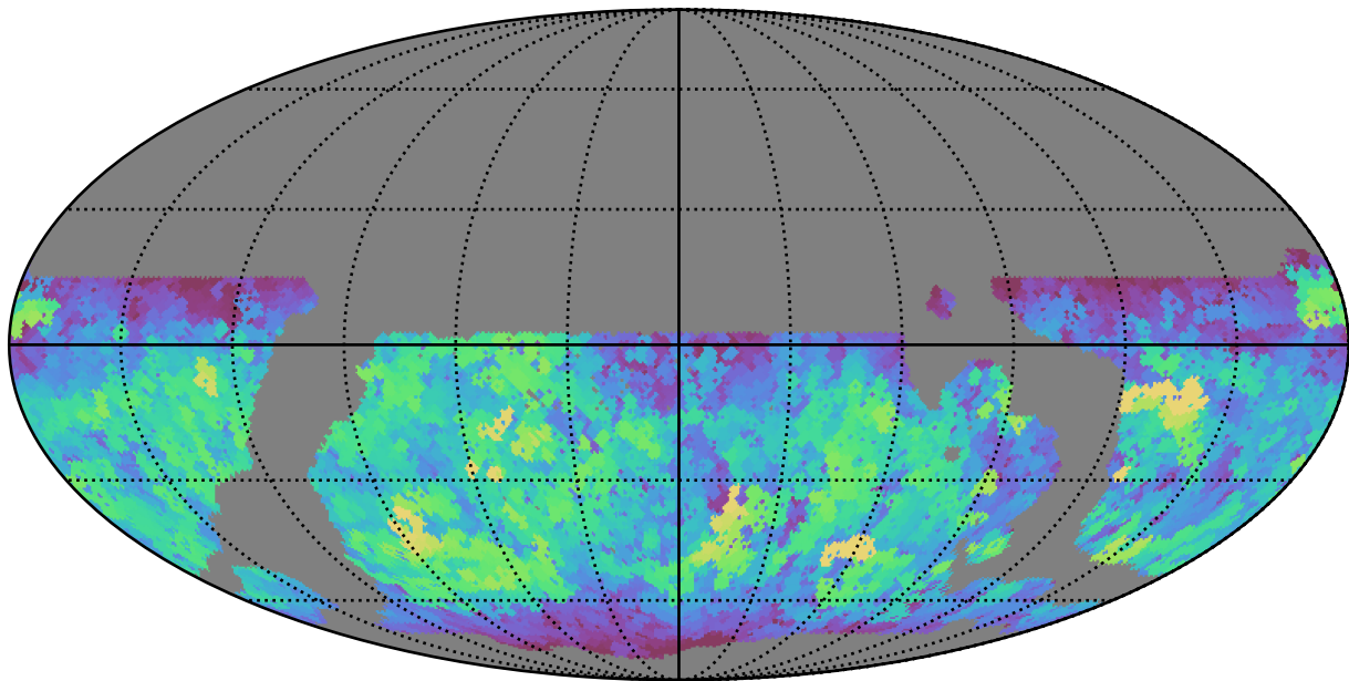
weather_cloudso35v3.4_10yrs WFD y band: Max saturation_mag
