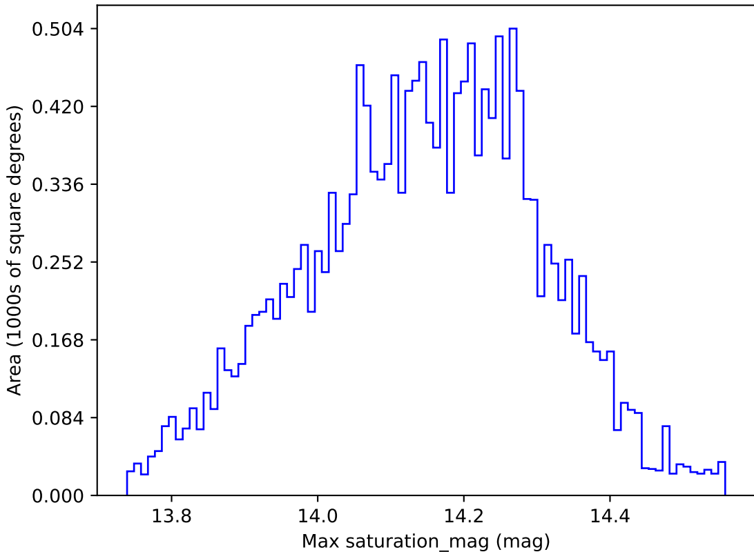
weather_cloudso35v3.4_10yrs WFD y band: Max saturation_mag
