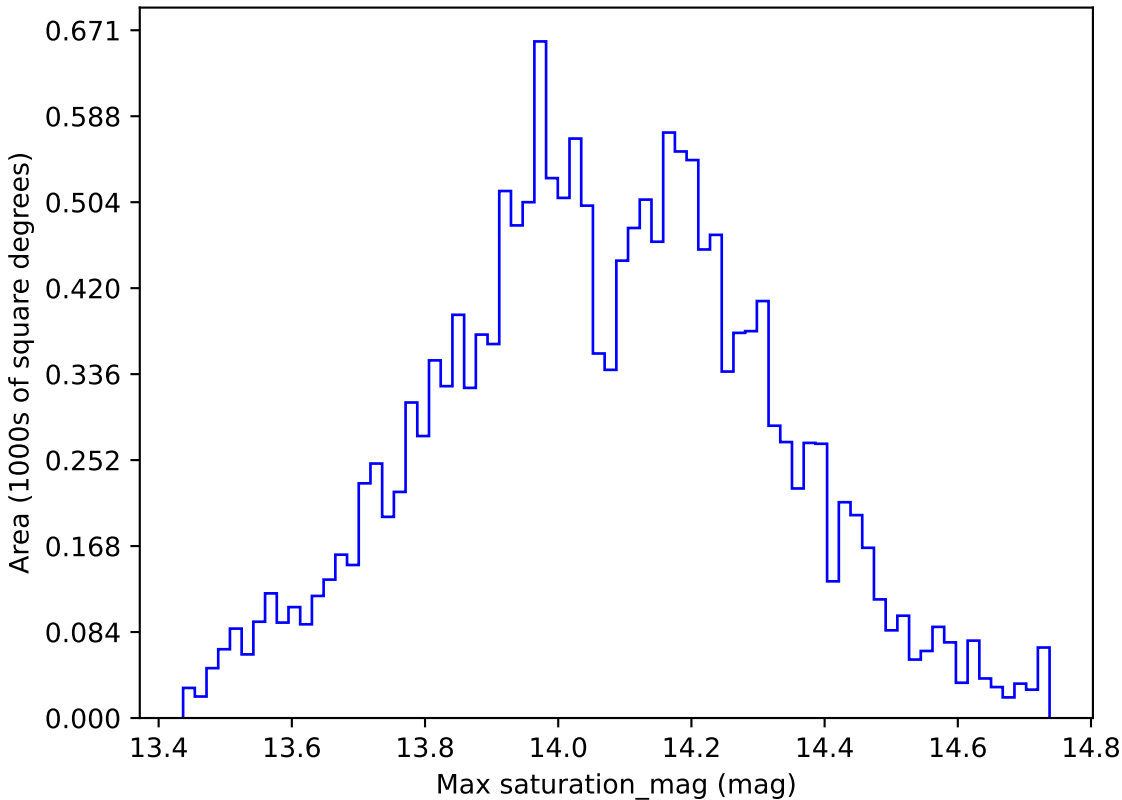
weather_cloudso35v3.4_10yrs WFD u band: Max saturation_mag
