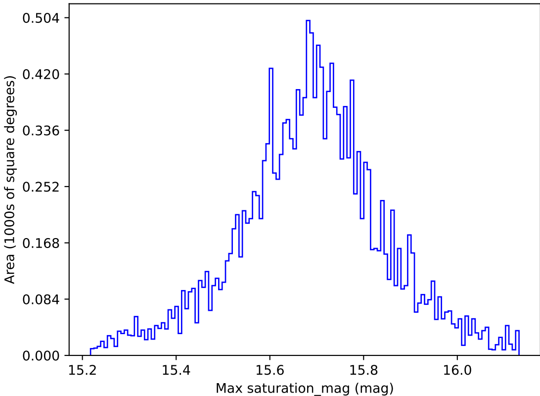
weather_cloudso35v3.4_10yrs WFD g band: Max saturation_mag
