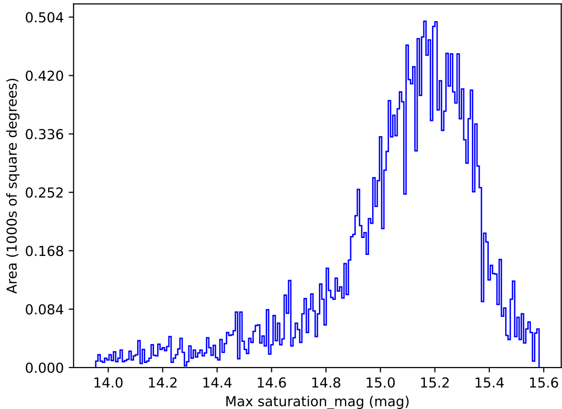
weather_cloudso35v3.4_10yrs All sky z band: Max saturation_mag
