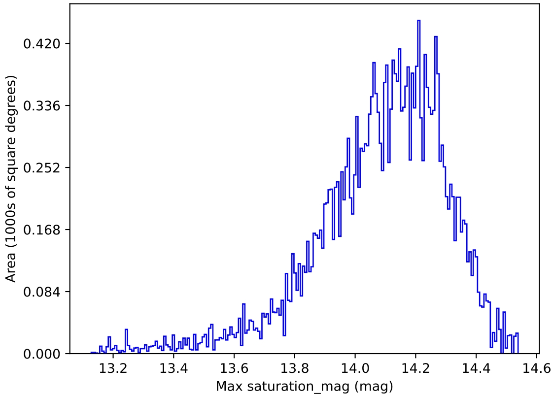
weather_cloudso35v3.4_10yrs All sky y band: Max saturation_mag
