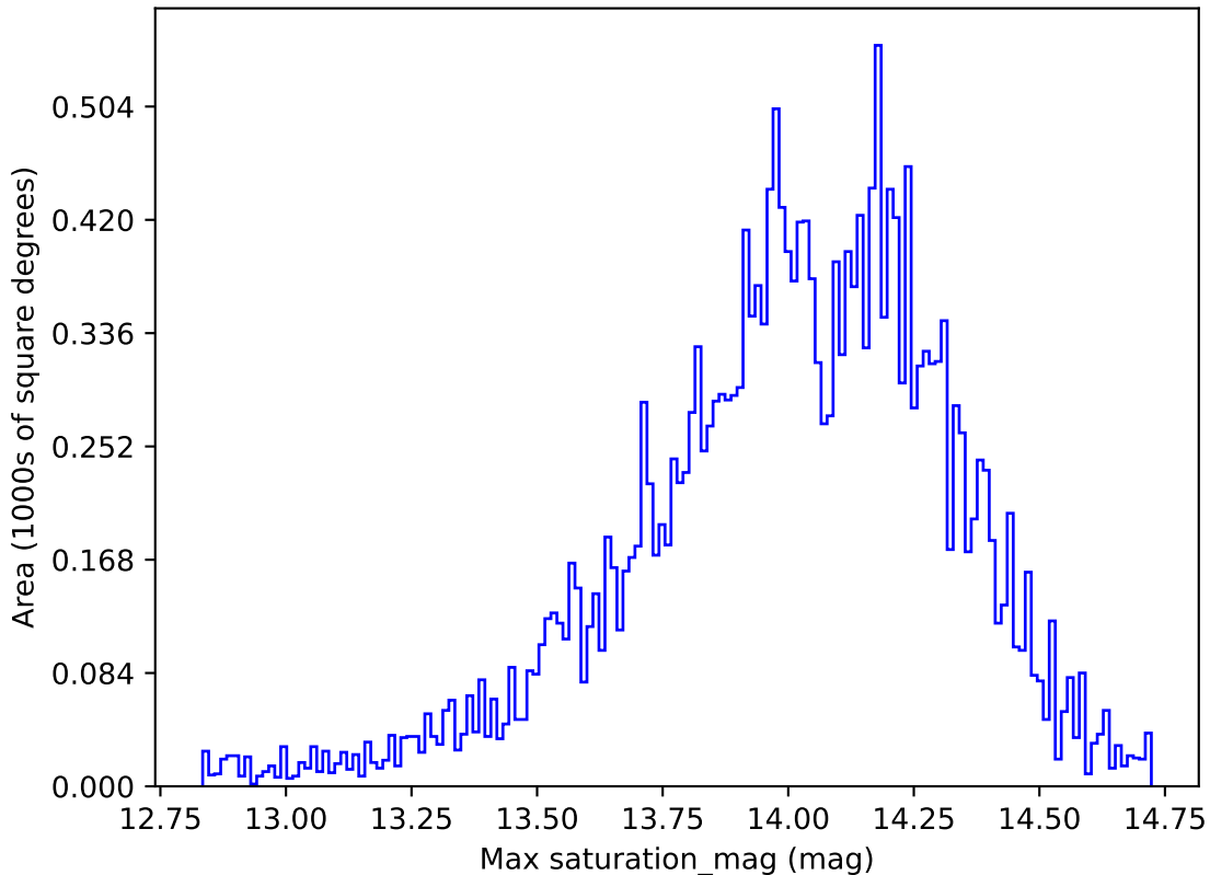
weather_cloudso35v3.4_10yrs All sky u band: Max saturation_mag
