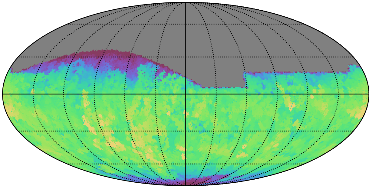
weather_cloudso35v3.4_10yrs All sky g band: Max saturation_mag
