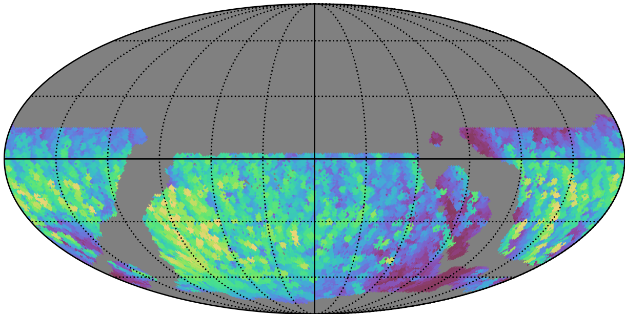
weather_cloudso35v3.4_10yrs WFD y band: Max normairmass
