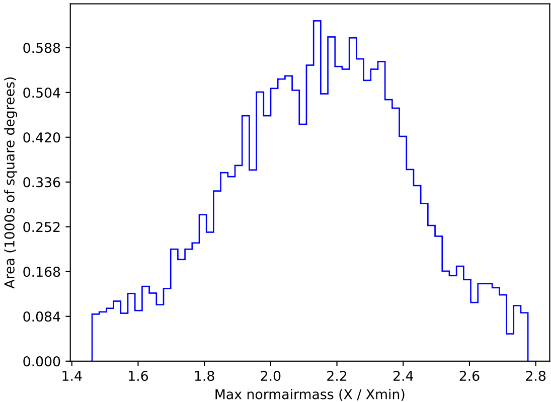
weather_cloudso35v3.4_10yrs WFD y band: Max normairmass
