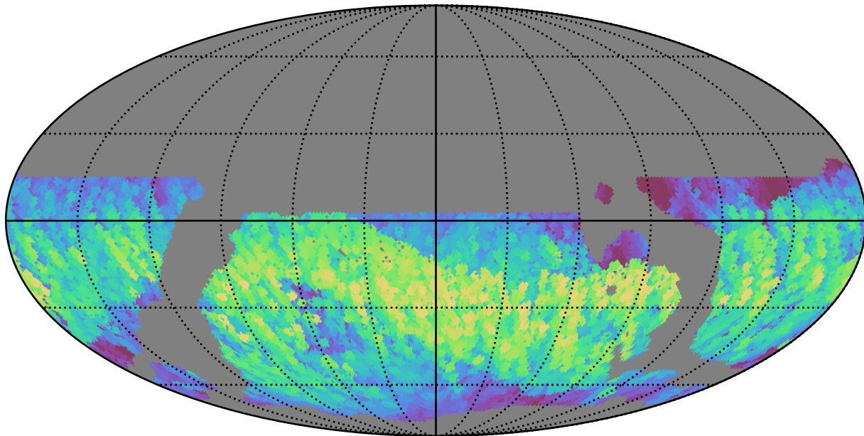
weather_cloudso35v3.4_10yrs WFD i band: Max normairmass
