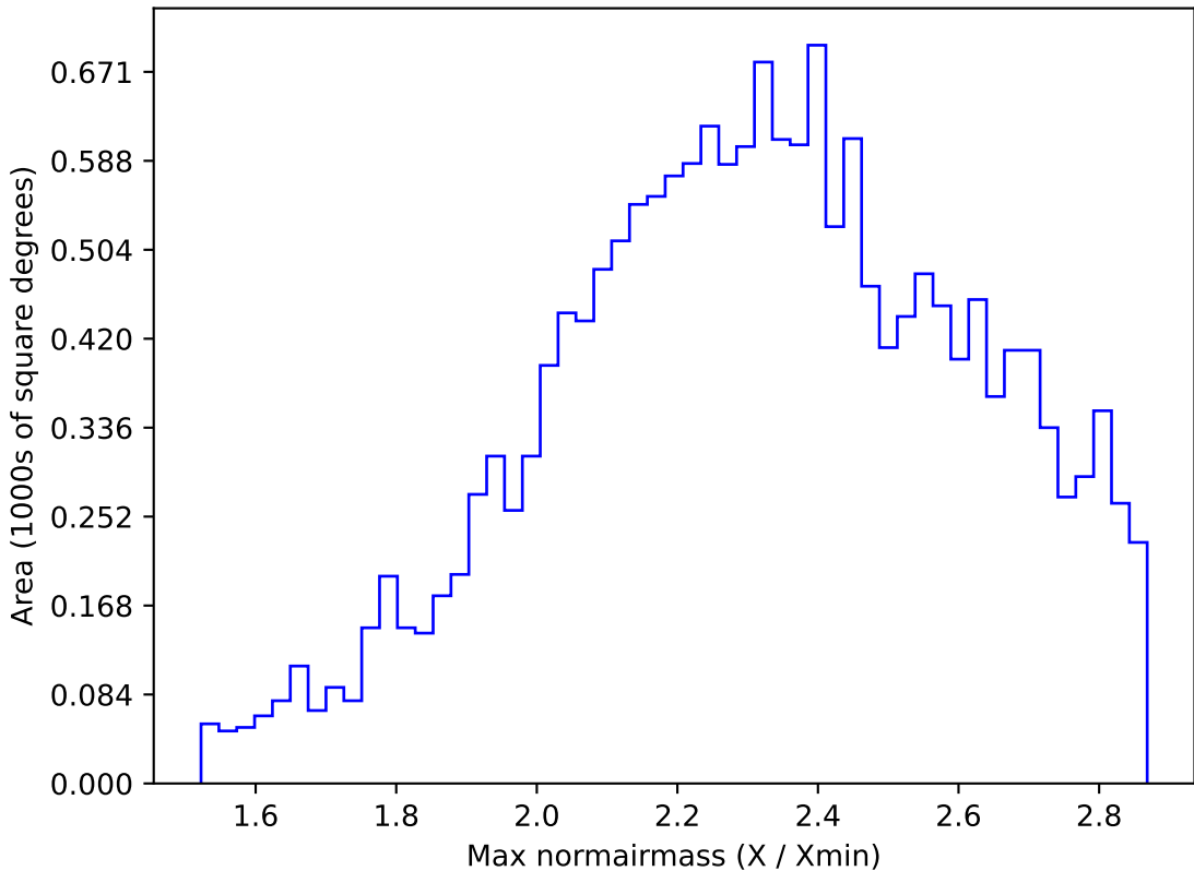
weather_cloudso35v3.4_10yrs WFD i band: Max normairmass
