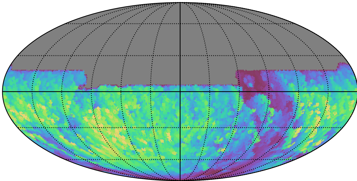
weather_cloudso35v3.4_10yrs All sky y band: Max normairmass
