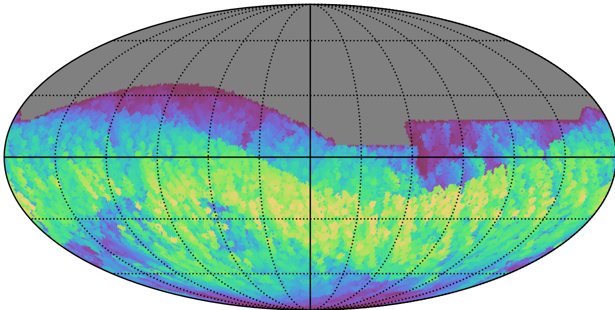
weather_cloudso35v3.4_10yrs All sky i band: Max normairmass
