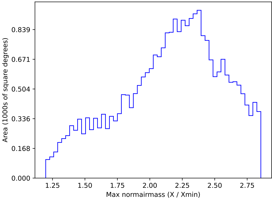
weather_cloudso35v3.4_10yrs All sky i band: Max normairmass
