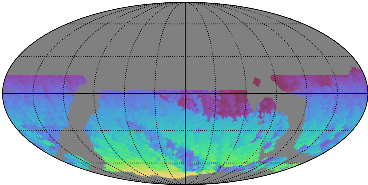
weather_cloudso35v3.4_10yrs WFD z band: Max HA
