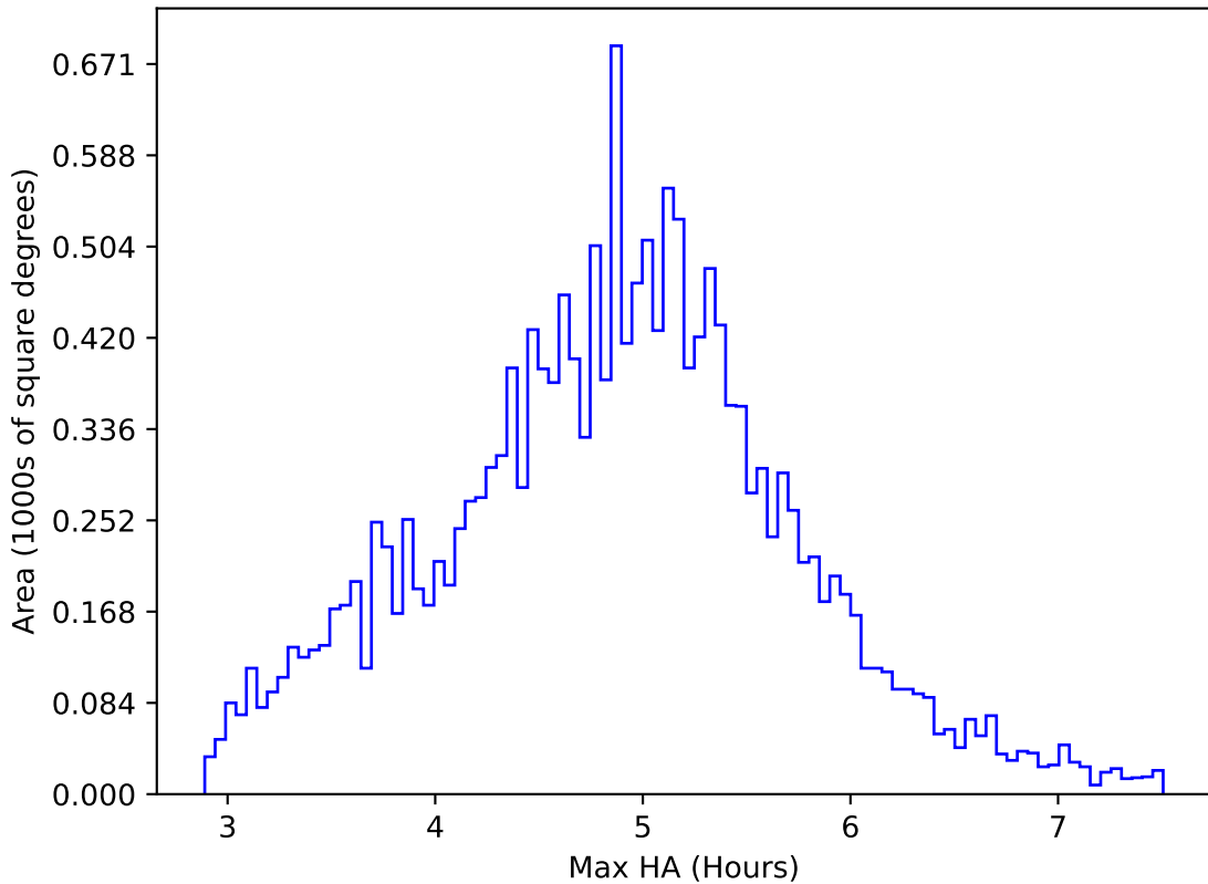
weather_cloudso35v3.4_10yrs WFD z band: Max HA
