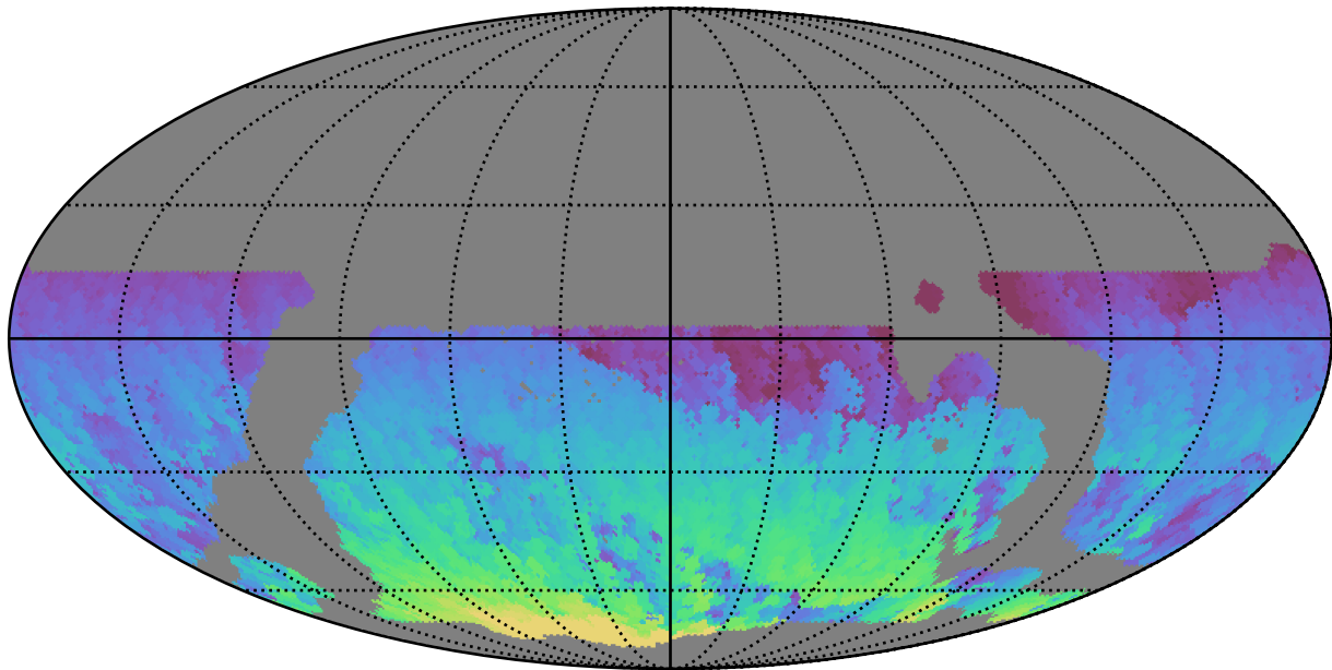
weather_cloudso35v3.4_10yrs WFD i band: Max HA
