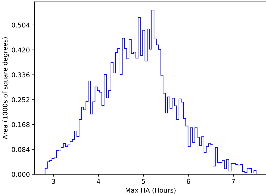
weather_cloudso35v3.4_10yrs WFD i band: Max HA
