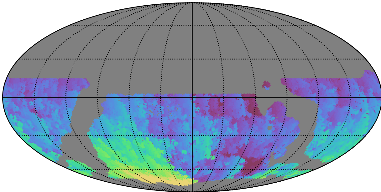
weather_cloudso35v3.4_10yrs WFD g band: Max HA
