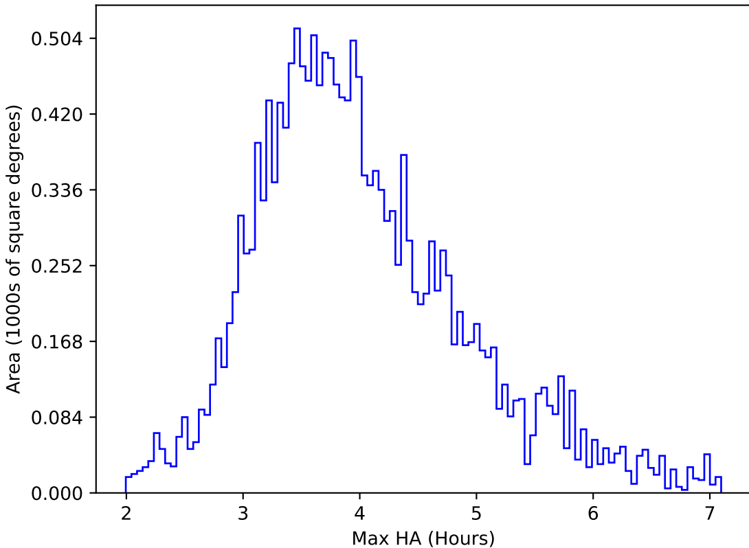
weather_cloudso35v3.4_10yrs WFD g band: Max HA
