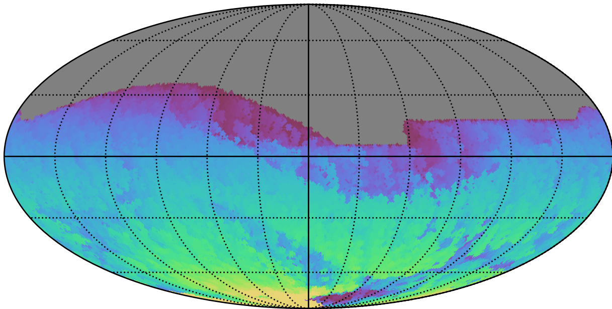
weather_cloudso35v3.4_10yrs All sky z band: Max HA
