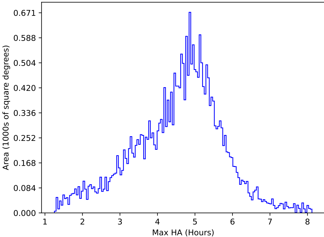
weather_cloudso35v3.4_10yrs All sky z band: Max HA
