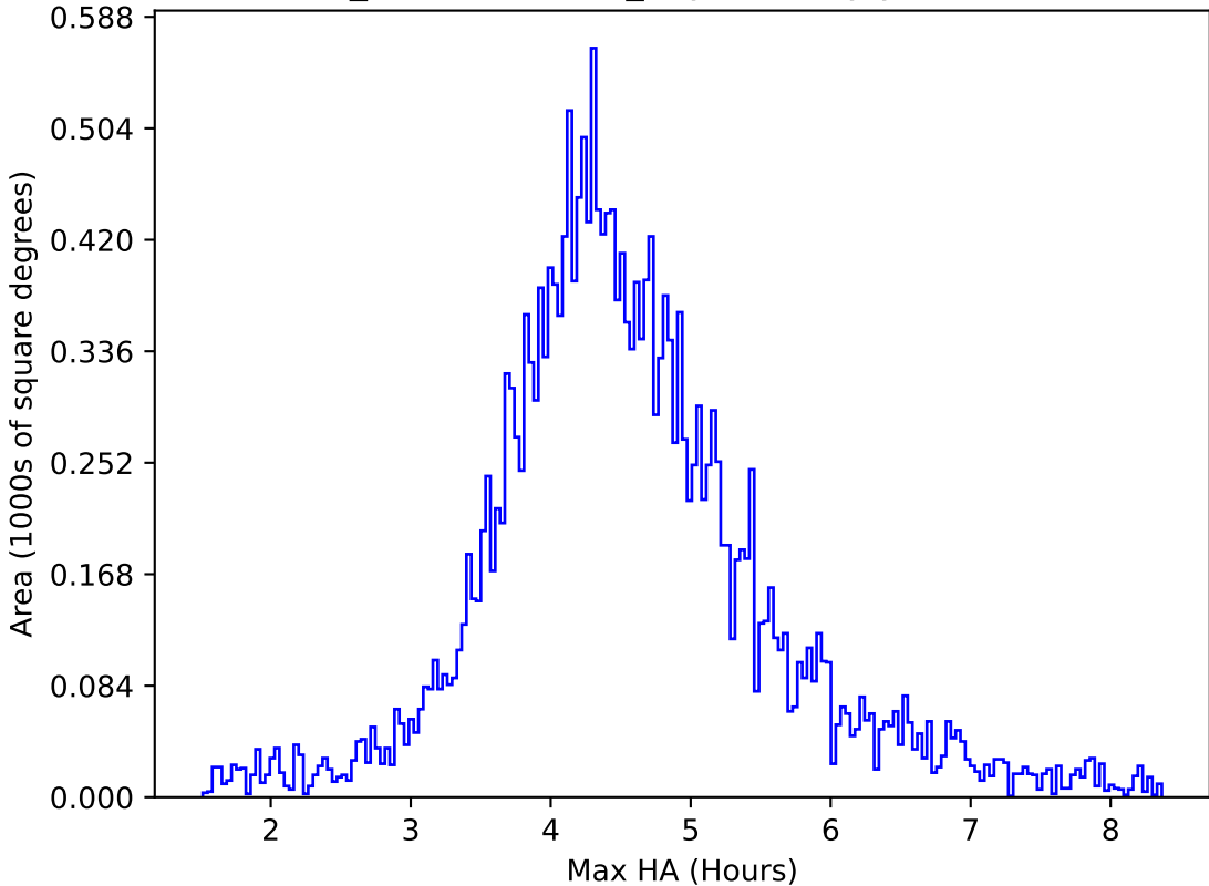
weather_cloudso35v3.4_10yrs All sky y band: Max HA
