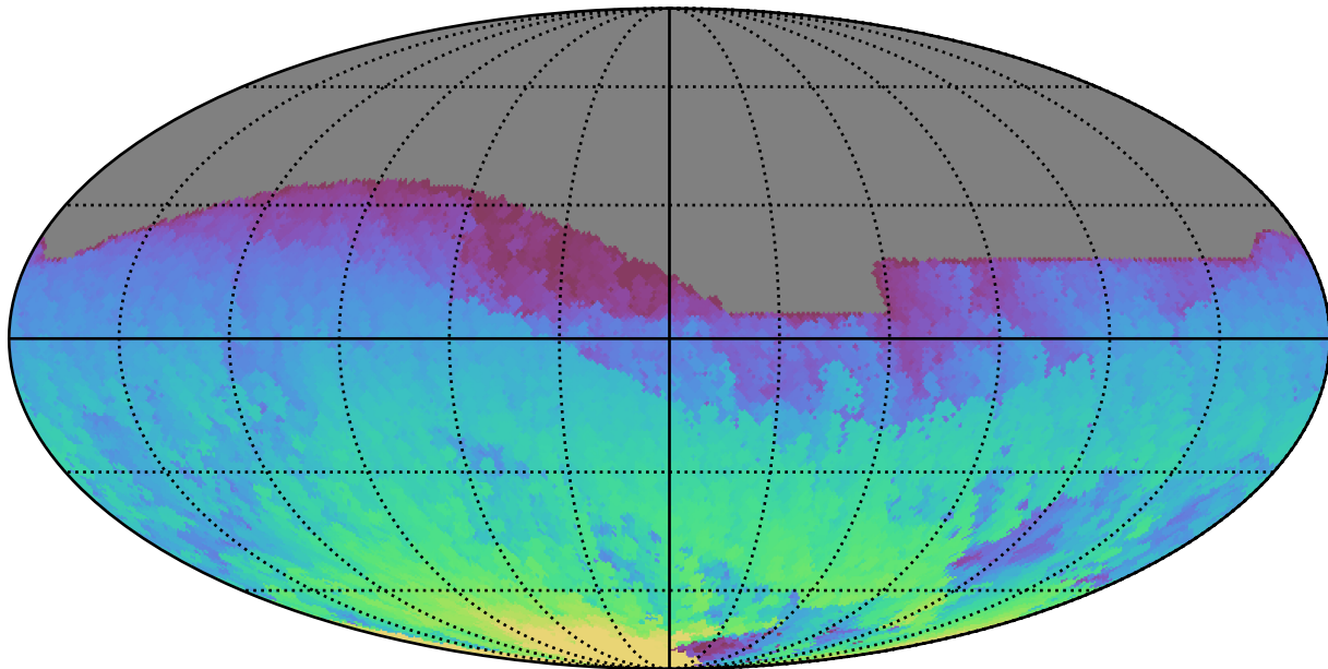
weather_cloudso35v3.4_10yrs All sky i band: Max HA
