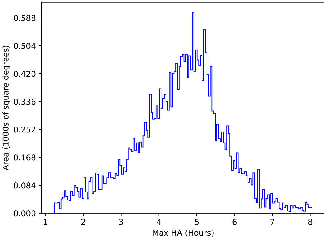
weather_cloudso35v3.4_10yrs All sky i band: Max HA
