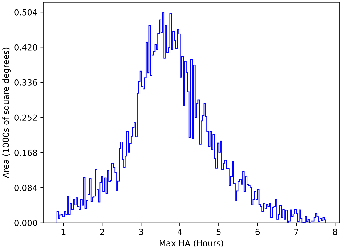
weather_cloudso35v3.4_10yrs All sky g band: Max HA
