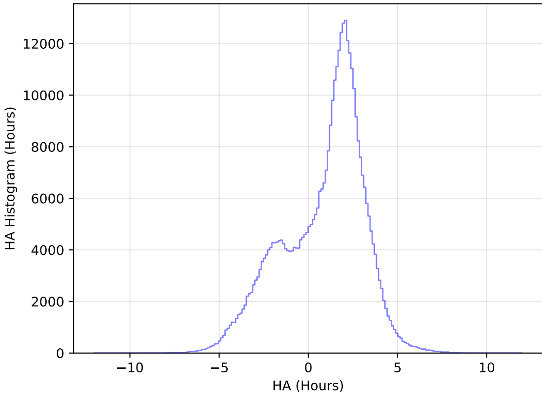
weather_cloudso35v3.4_10yrs WFD y band: HA Histogram
