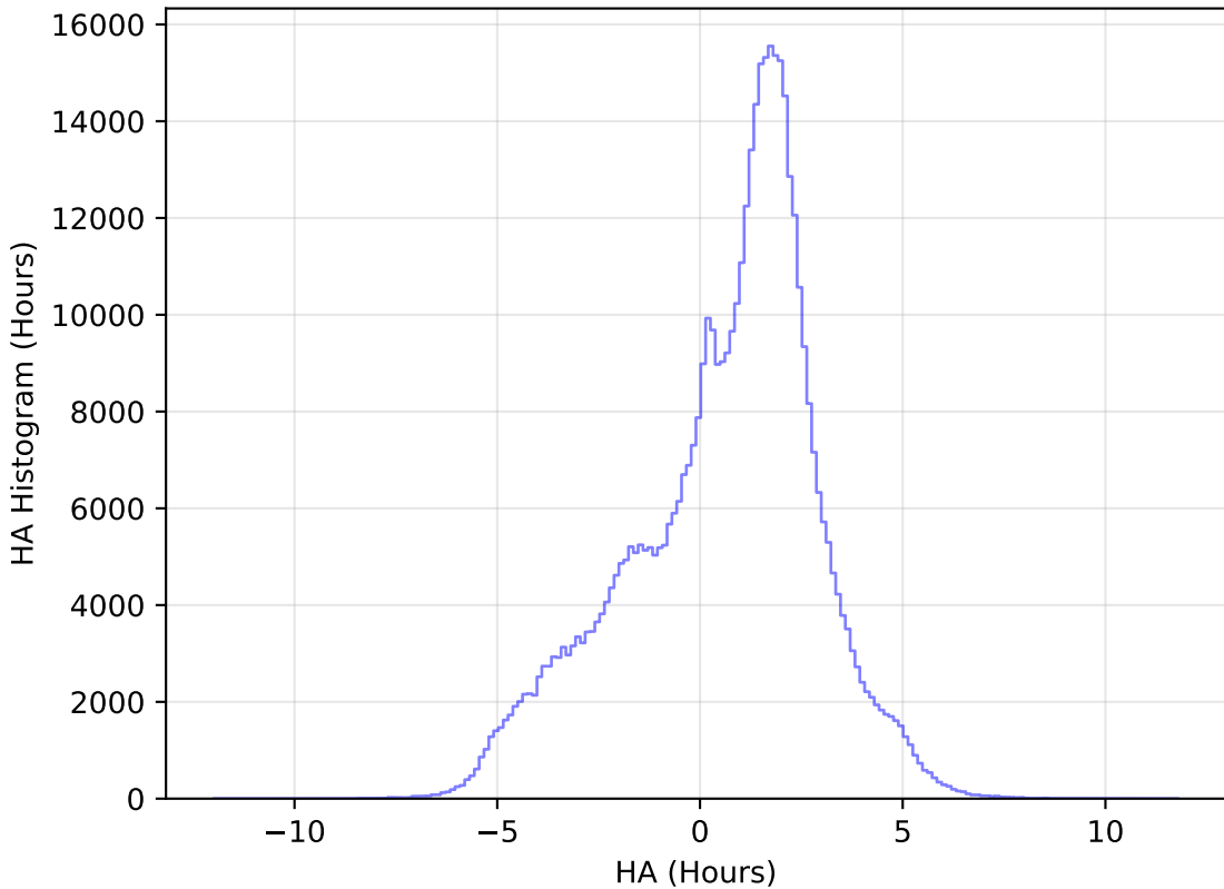
weather_cloudso35v3.4_10yrs WFD i band: HA Histogram
