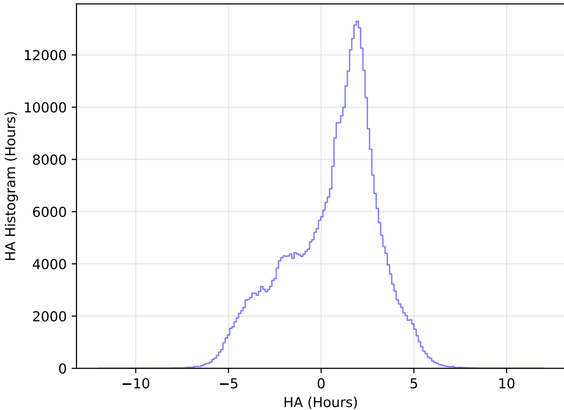
weather_cloudso35v3.4_10yrs All sky z band: HA Histogram
