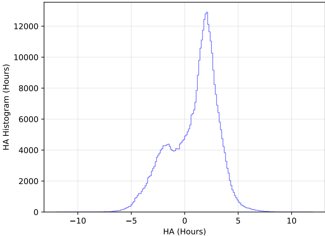
weather_cloudso35v3.4_10yrs All sky y band: HA Histogram
